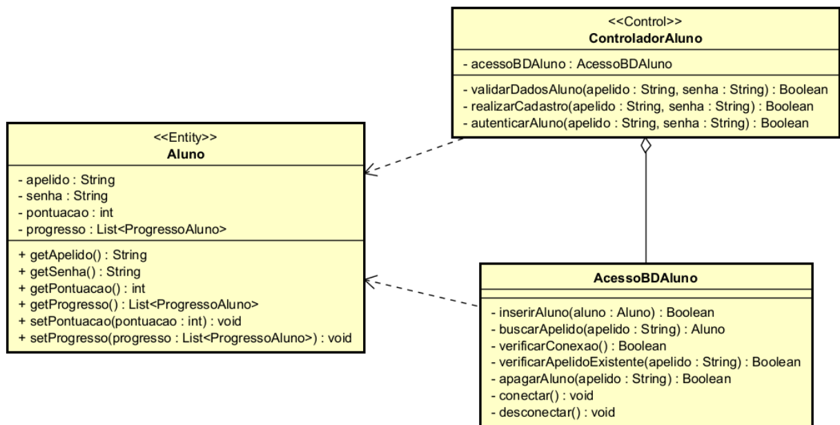
Diagrama de Clases para CSU02 e CSU03
